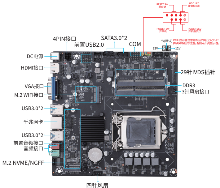
图1-1 H311M-I 主板图解
